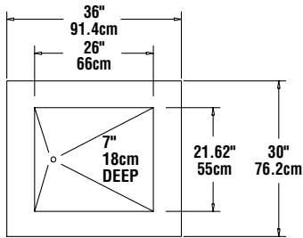
PLAN VIEW KCI-36/ KCI-36-NU
