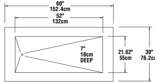
PLAN VIEW KCI-60/ KCI-60-NU
