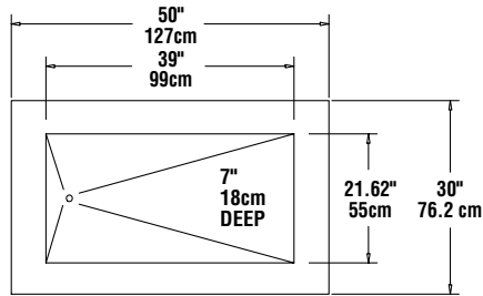
PLAN VIEW KCI-50/ KCI-50-NU
