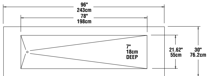
PLAN VIEW KCI-96/ KCI-96-NU
