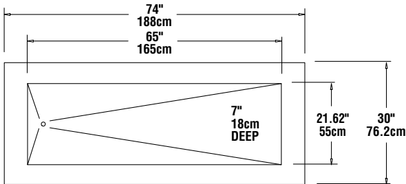
PLAN VIEW KCI-74/ KCI-74-NU
